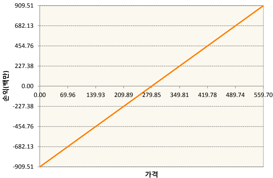
KR4101Q90009-2020-09 코스피200지수선물
