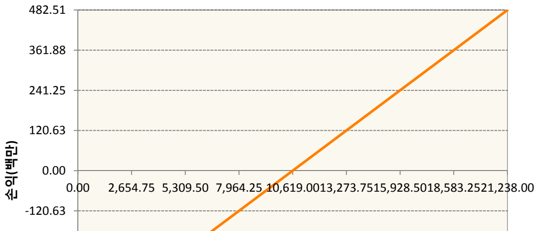
HCG0-HSCEI Futures Feb20
