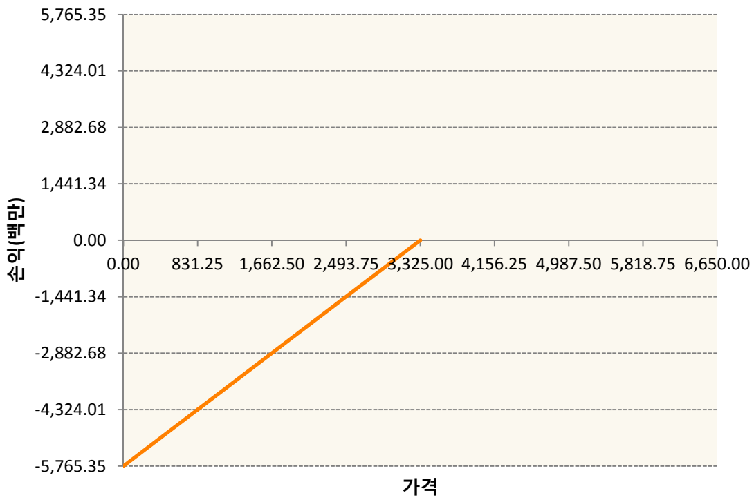
OESXU9-P3325-EURO STOXX 50
