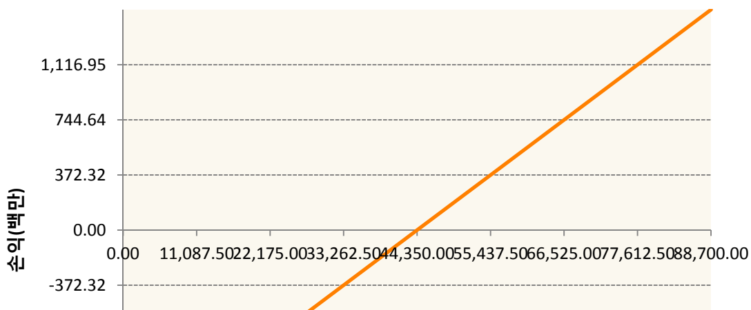
KR4111P90000-2019-09 삼성전자개별선물
