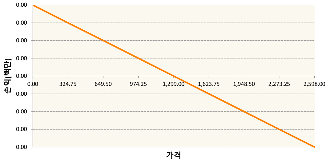
KR4175T30003-2023-03 달러선물
