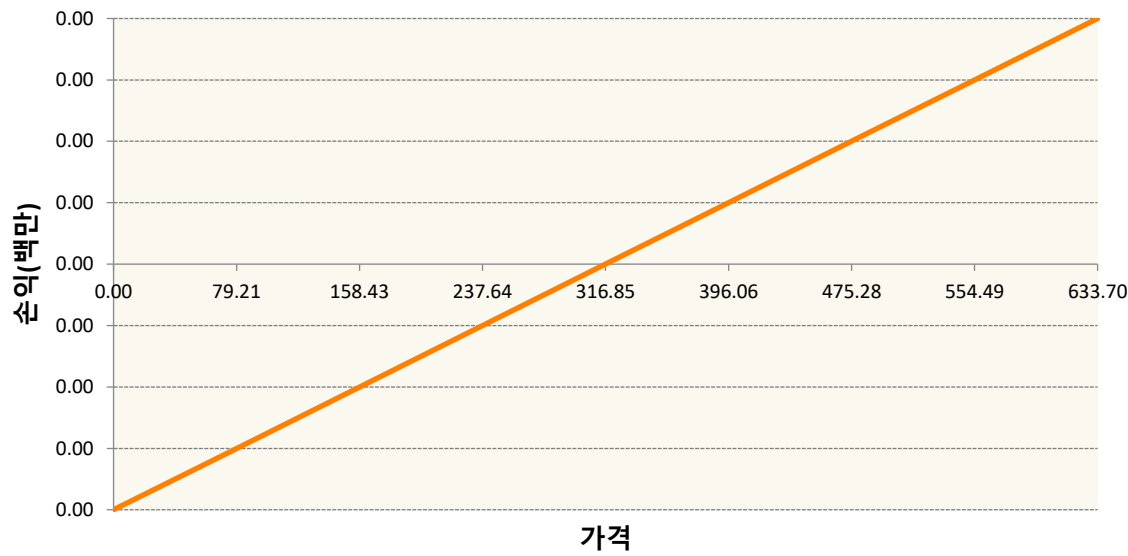
KR4101T30009-2023-03 코스피200지수선물
