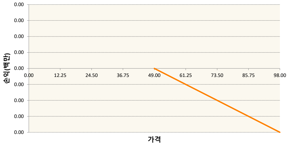
OESXU2-C3725-EURO STOXX 50
