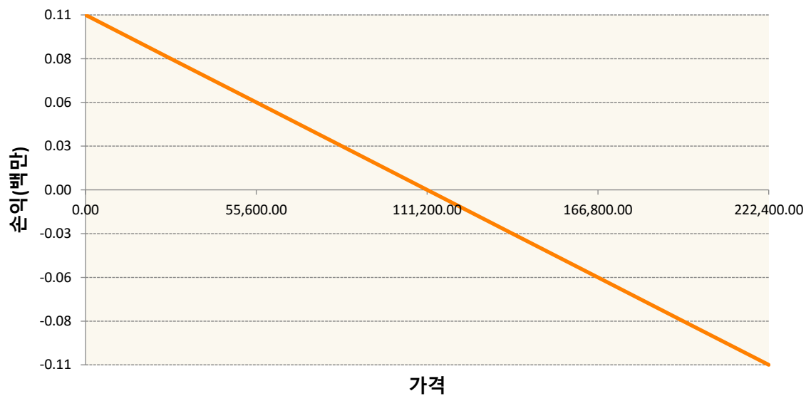
KR41EYS80008-2022-08 에코프로비엠개별선물
