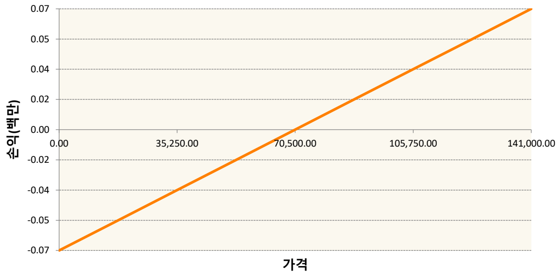
KR41CFS80001-2022-08 카카오개별선물
