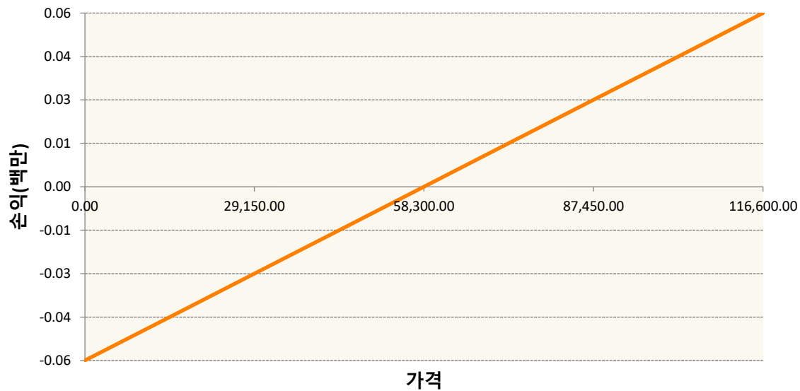
KR4111S80005-2022-08 삼성전자개별선물
