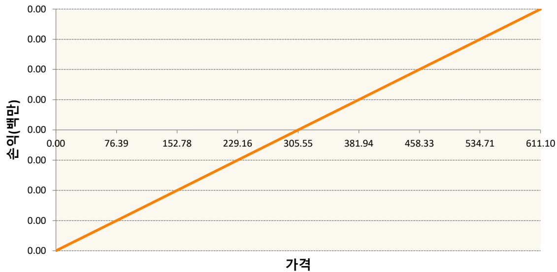
KR4101S90005-2022-09 코스피200지수선물
